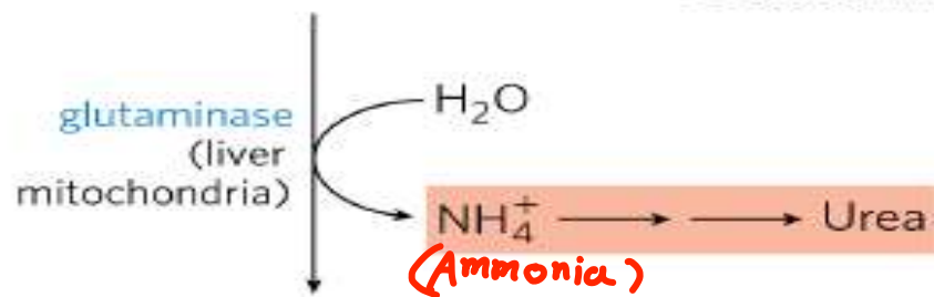
L-Glutamine
